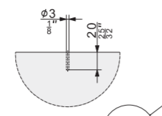
DETAIL G 2:1
