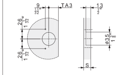
DETAIL F 2:1
