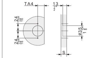
DETAIL E 2:1
