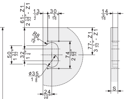
DETAIL D 2:1
